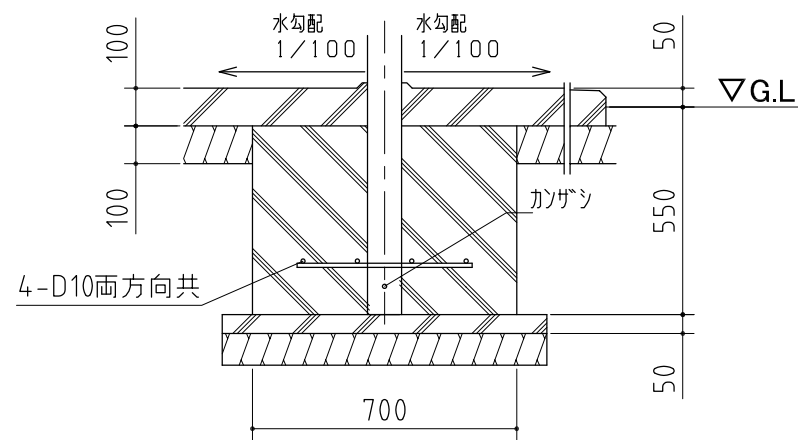
A-A' 断面 1/20
